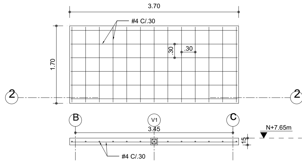
DETALLE PLACA DE TANQUES ESCALA 1:50
