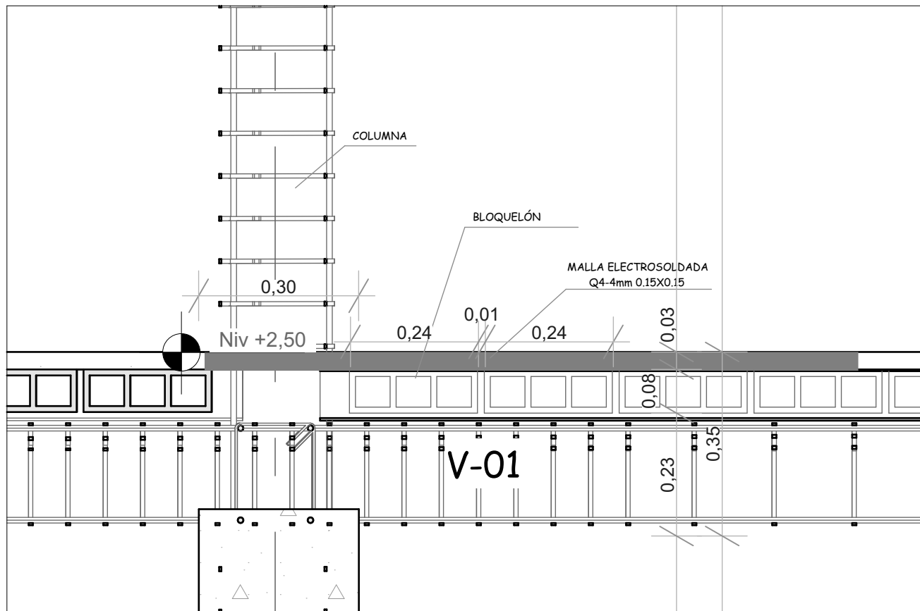
DETALLE DE ENTREPISO Esc 1: 10
