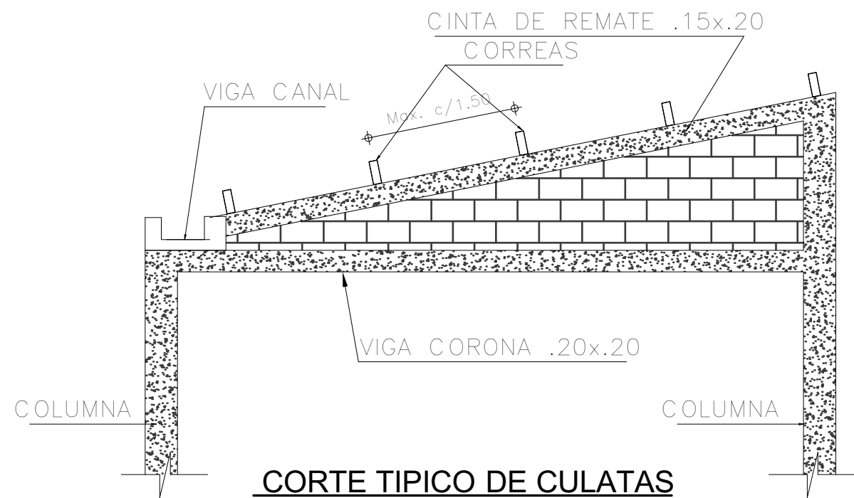
CORTE TIPOICO DE CULATAS Esc. 1 : 5 0
