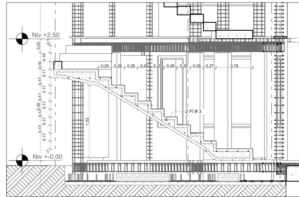
ALZADO DE ESCALERA Esc 1: 50
