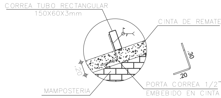
DETALLE DE CORREA Esc. 1 : 2 5
