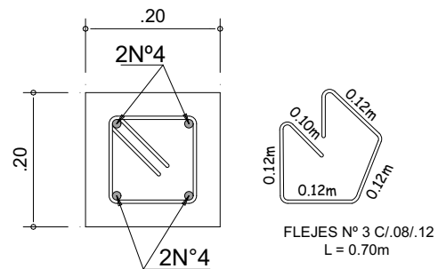
DETALLE VIGA CUBIERTA (VCU-20x20)
