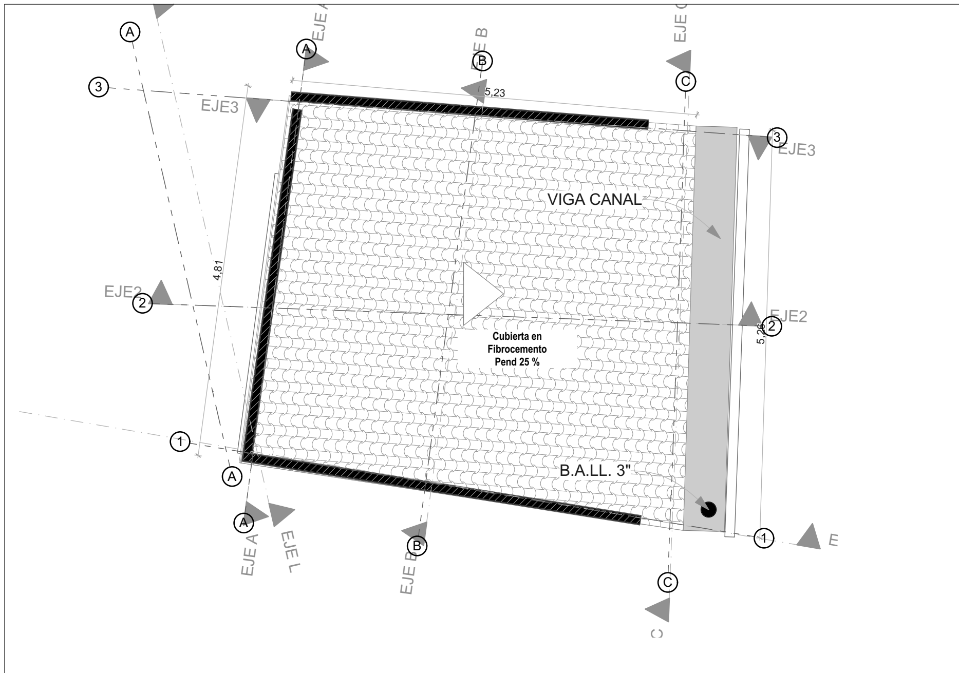
Planta de Cubierta Esc 1: 50
